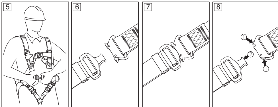
Регулирование набедренных лямок и ремней предохранительного пояса
